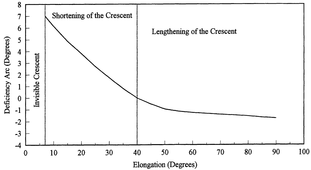
FIG. 2 Danjon limit.
