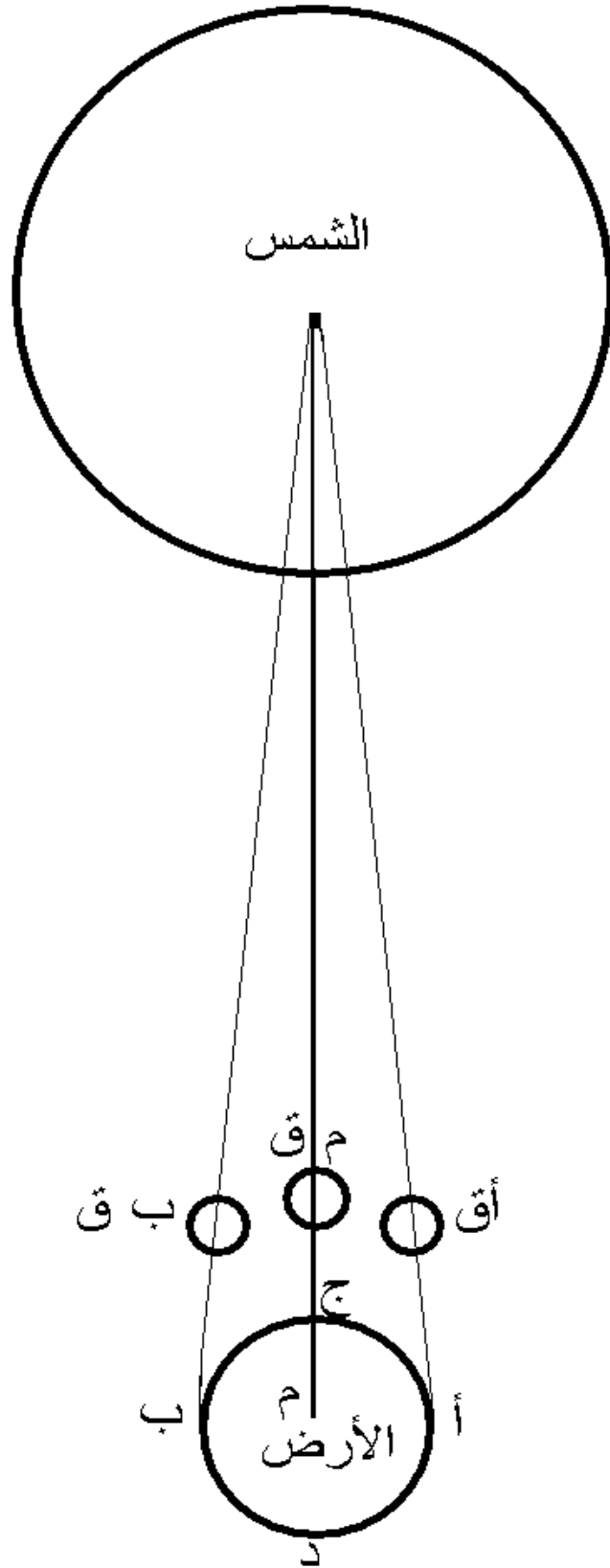
الشكل رقم (2): يبين هذا الشكل مواقع القمر المختلفة عند حدوث الاقتران المركزي و الاقتران السطحي من عدة مواقع على سطح الكرة الأرضية. نسب الأبعاد ليست حسب الواقع.
